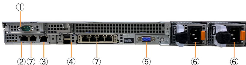
図 2-7. Deep Discovery Inspector 1300 の背面パネル
