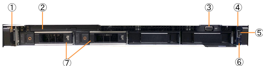
図 2-3. Deep Discovery Inspector 1300 の前面パネル
