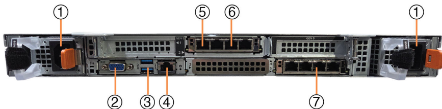
図 2-6. Deep Discovery Inspector 550/1500 の背面パネル
