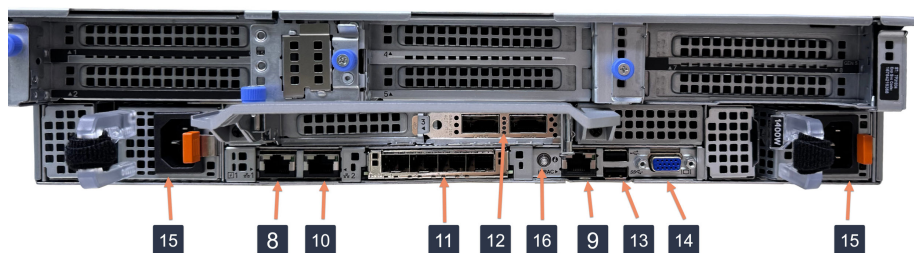
図 2-9. Deep Discovery Inspector 40G の背面パネル
