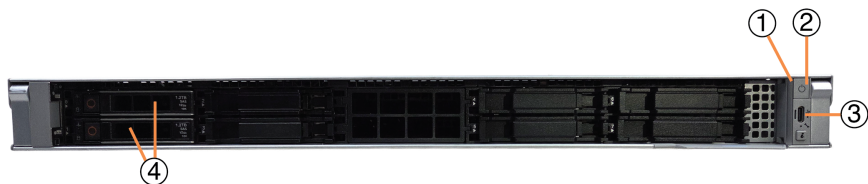
図 2-2. Deep Discovery Inspector 550/1500 の前面パネル
