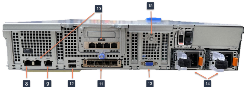
図 2-8. Deep Discovery Inspector 4300/9300 の背面パネル
