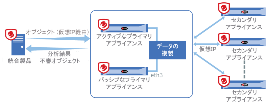
図 2-3. 負荷分散機能を備えた高可用性クラスター
