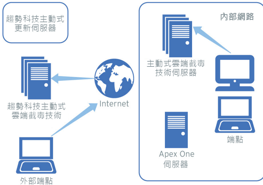
圖 4-2. 查詢程序
