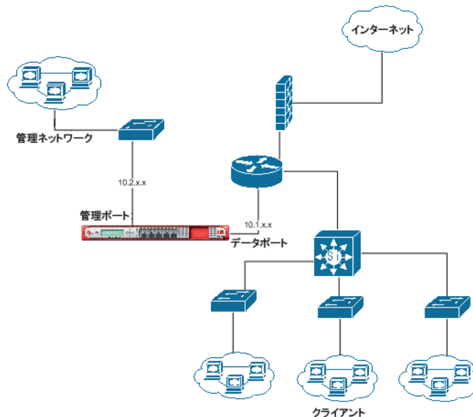
図 15-11. ネットワーク内での IWSVA 管理インターフェースの配置
