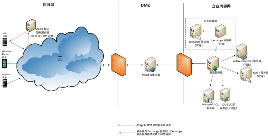
图 1-2. 包含本地通信服务器的增强安全型号
