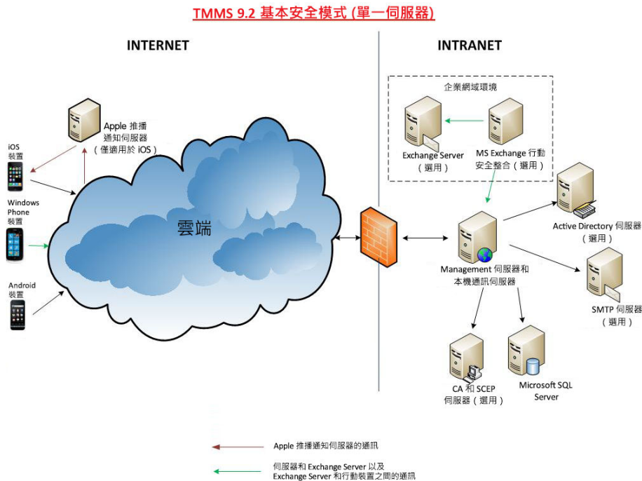
圖 1-3. 基本安全模式
