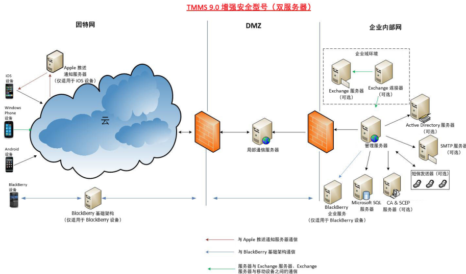
图 1-2. 包含本地通信服务器的增强安全型号
