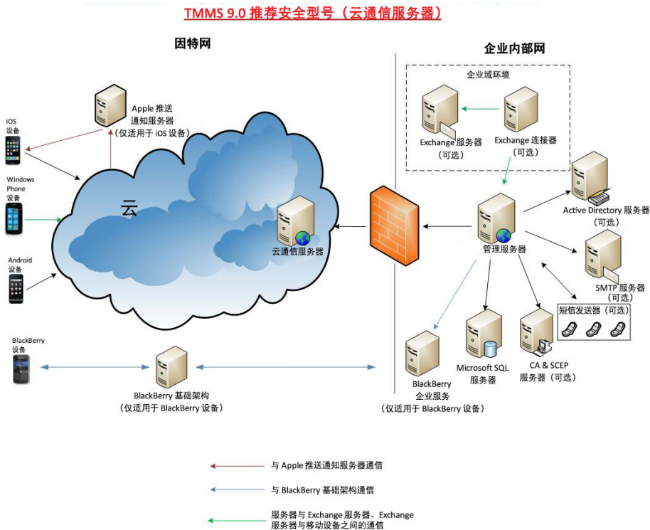
图 1-1. 包含云通信服务器的增强安全型号
